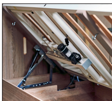
Elektrisk hovedgærde
