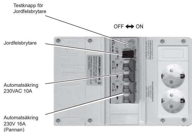
Elboxens baksida
