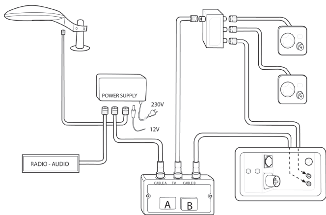
Schematisk illustration av antensystemet.
