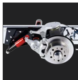
Luftfjädring AL-KO (bak) 780, i760, i810 X2 tvåaxling 880, i860, i910 X2 treaxling i810 Tandem X2 treaxling
