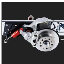
Luftfjädring AL-KO (fram/bak) 780, i760, i810 X4 tvåaxling 880, i860, i910 X4 treaxling i810 Tandem X4 treaxling
