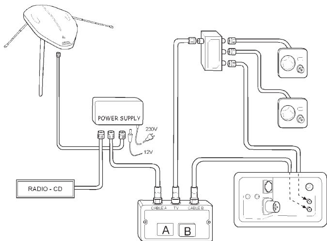
Schematisk illustration av antenssystemet.
