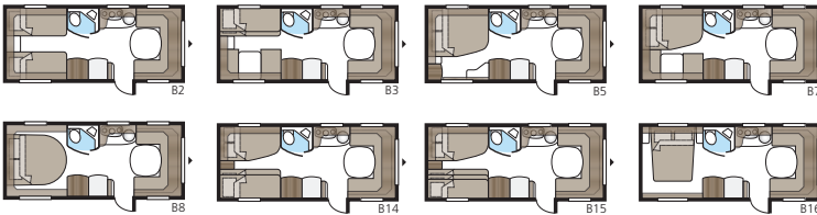
Planlösningar
