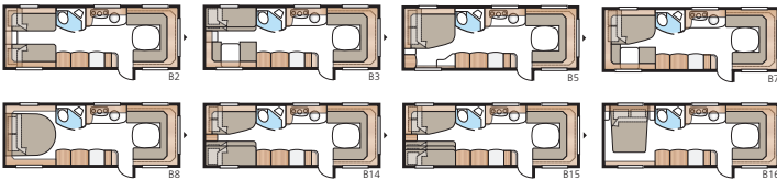
Planlösningar
