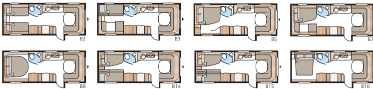
Planlösningar
