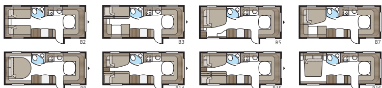
Planlösningar
