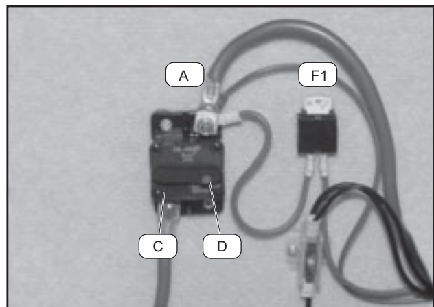
Komponenter som kopplar samman 12V-systemen.
