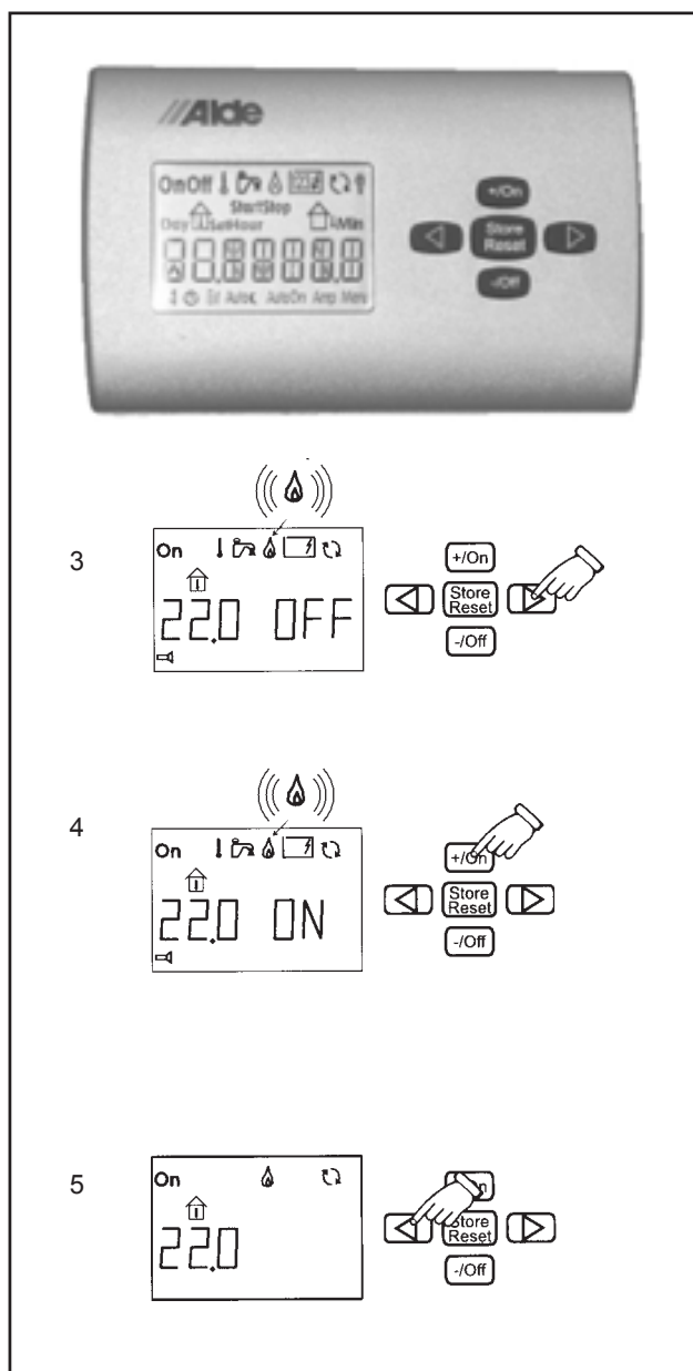
Värmepannans manöverpanel.
