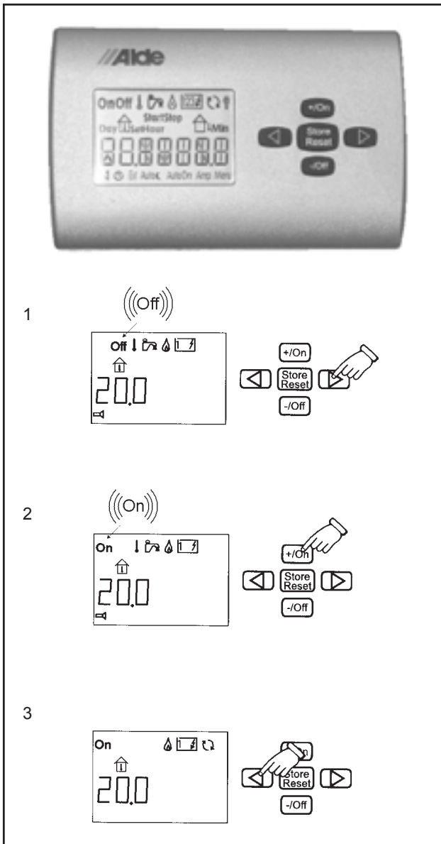
Värmepannans manöverpanel.
