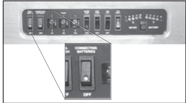
Strömbrytare "CONNECTING BATTERIES" för att koppla samman bodelens och bilens 12V-systemen.
