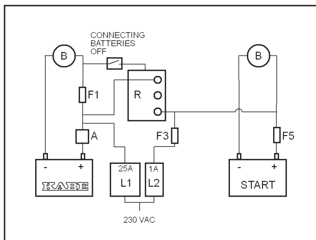
Schematisk illustration av hur bodelens batteri och bilens startbatteri är kopplat till batteriladdare L1 och L2. B illustrerar övriga elektriska belastningar i resp system.
