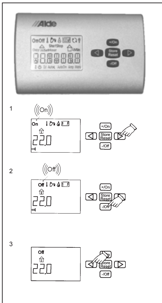
Värmepannans manöverpanel.
