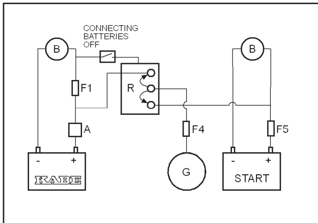
Laddströmsfördelaren (R)
